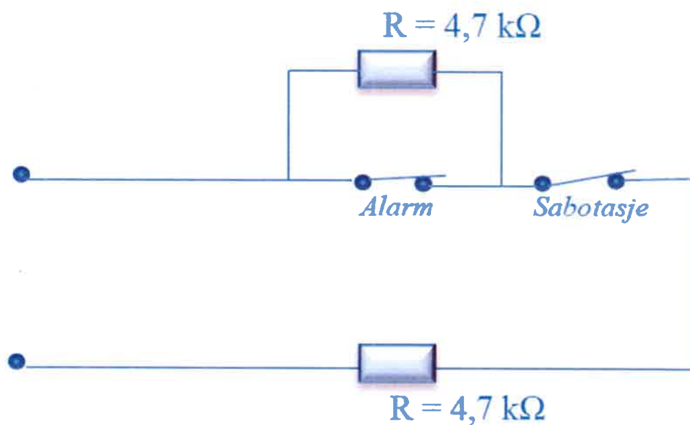
Figur 4.13 Dobbelt-balansert alarmsløyfeprinsipp
