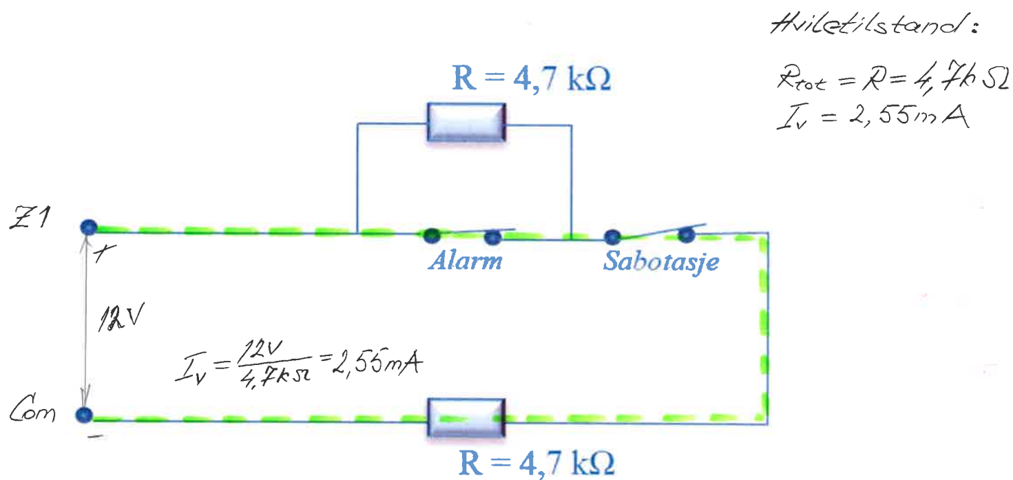
Figur 4.13 Dobbelt-balansert alarmsløyfeprinsipp
