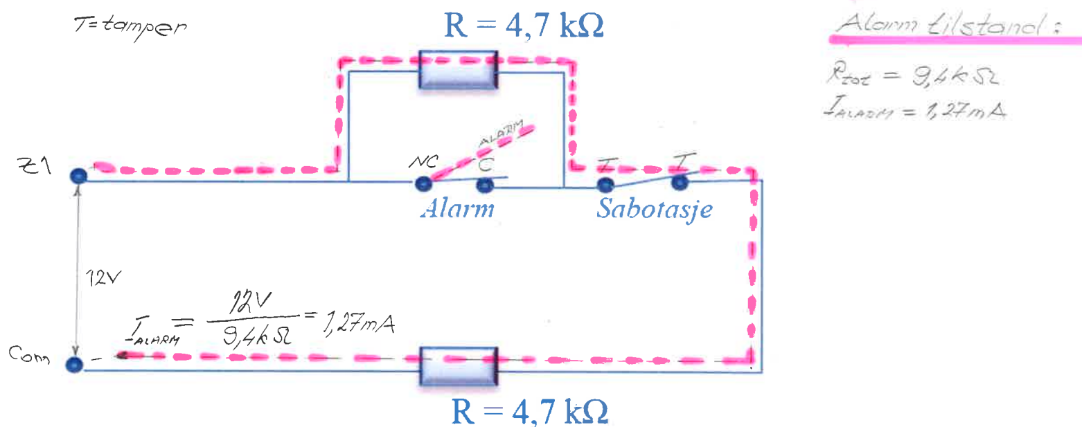
Figur 4.13 Dobbelt-balansert alarmsløyfeprinsipp
